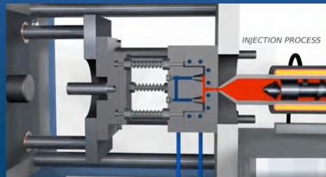
注塑成形
