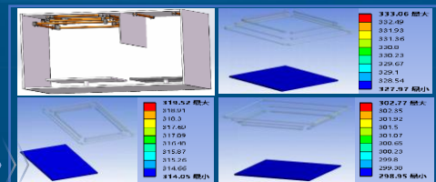
独立控温，预热温度场仿真分析
