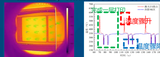
检测温度分布及历程
