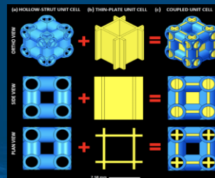
可打印复杂结构
