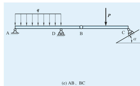
题 1-2 图
