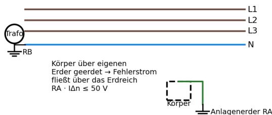
TT-System (Anlagenerder, RCD nötig)
