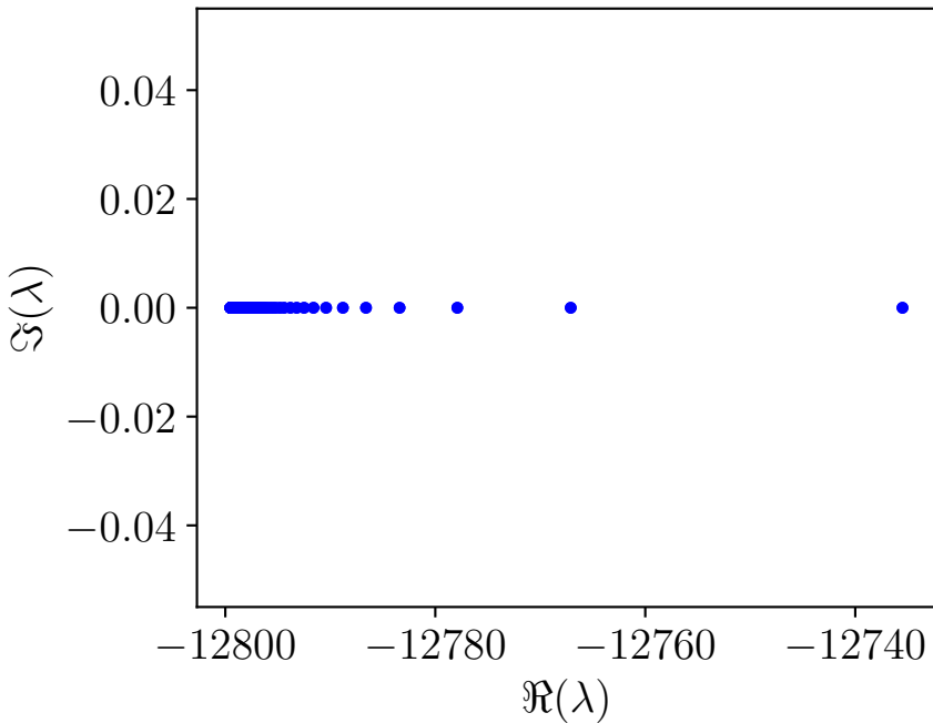
diffusion \lambda_{max}
