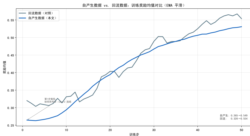
图 6.4 自产生数据（本文）与回流数据（对照）训练的奖励均值对比（EMA 平滑）
