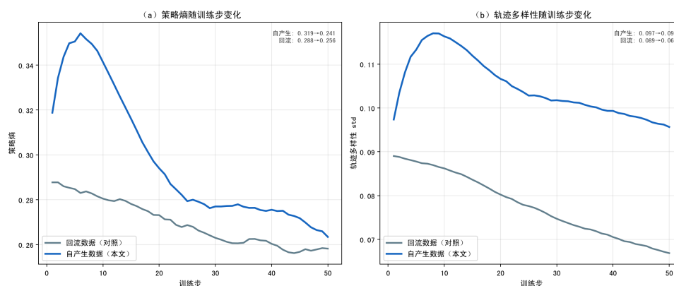
图 6.6 策略熵与轨迹多样性 std 随训练步的变化（EMA 平滑）
