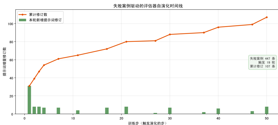
图 6.5 失败案例驱动的评估器自演化时间线
