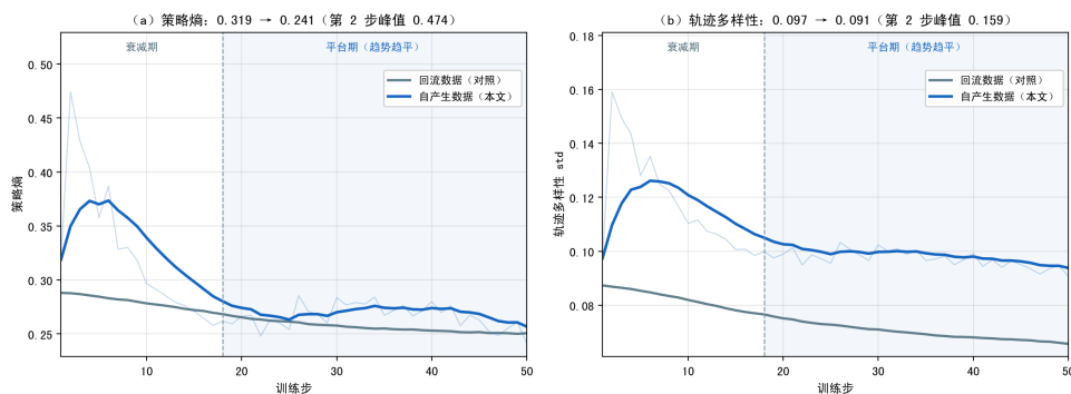
图 5.5 策略熵与轨迹多样性 std 随训练步的变化（EMA 平滑）
