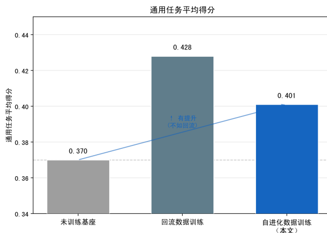
图 5.7 三个模型在通用任务上的平均得分
