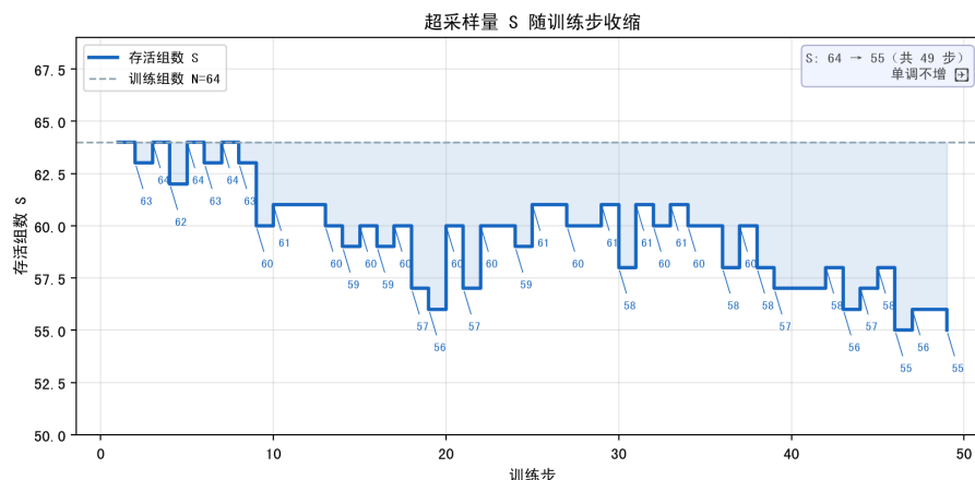
图 6.1 超采样量 S 随训练步收缩
