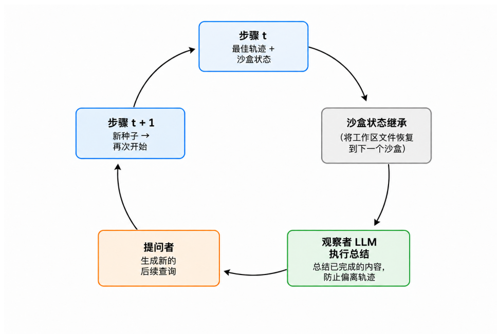
图 4.3 跨步自进化闭环
