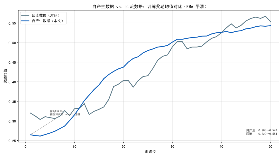
图 5.3 自产生数据（本文）与回流数据（对照）训练的奖励均值对比（EMA 平滑）
