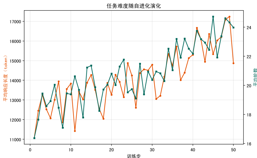
图 5.2 任务难度随自进化演化：平均响应长度与交互轮数
