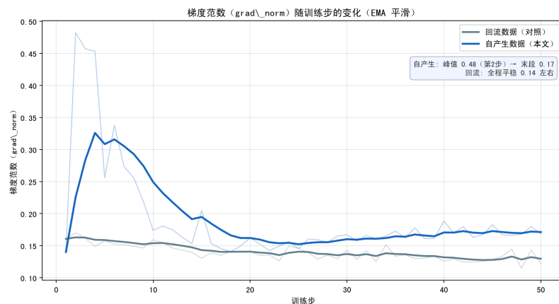
图 5.6 梯度范数 (grad_norm) 随训练步的变化
