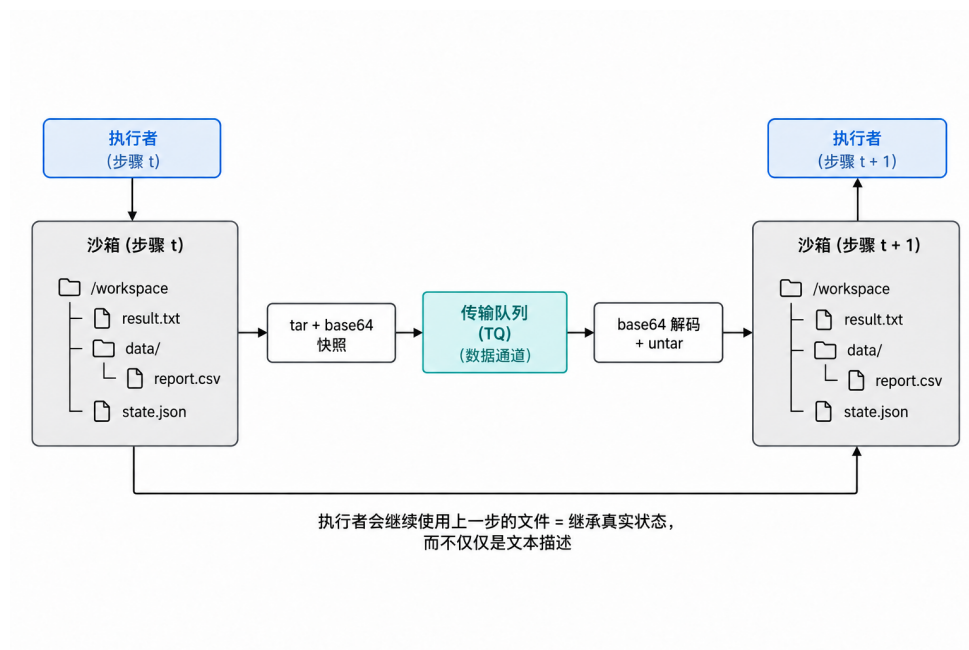
图 4.4 沙箱状态继承机制
