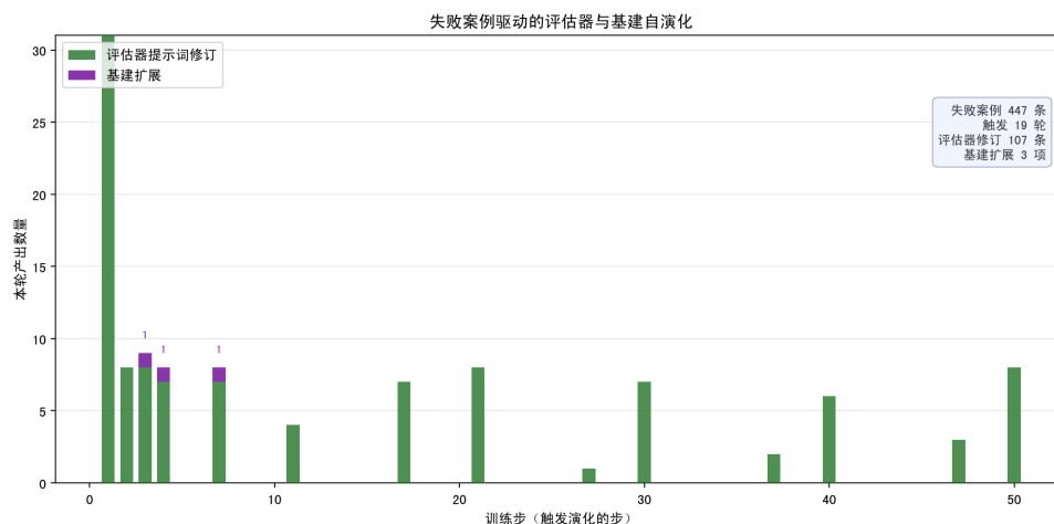
图 5.4 失败案例驱动的评价器与基建自演化时间线
