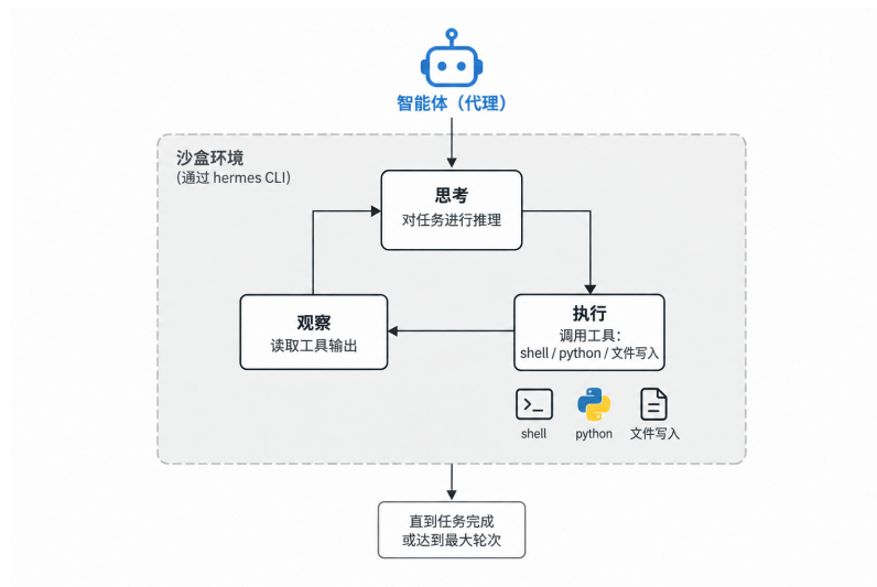
图 4.12 执行者沙箱内 ReAct 循环
