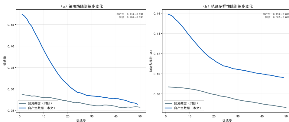
图 5.5 策略熵与轨迹多样性 std 随训练步的变化（EMA 平滑）
