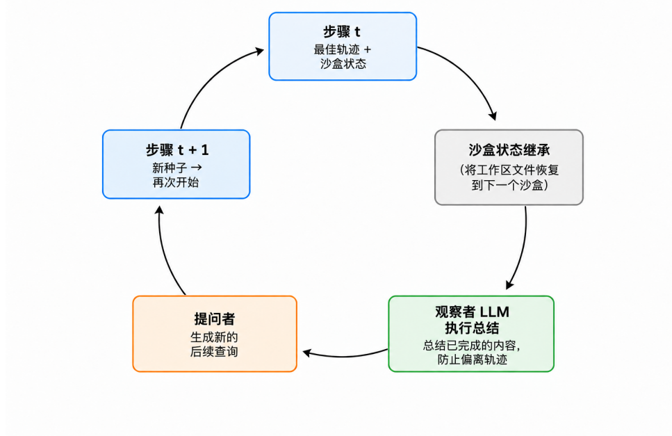
图 4.3 跨步自进化闭环
