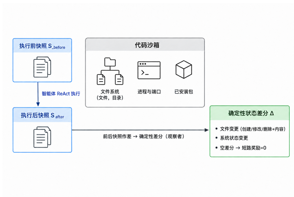
图 4.6 沙箱环境与状态管理：执行前后快照作差得到确定性状态差分
