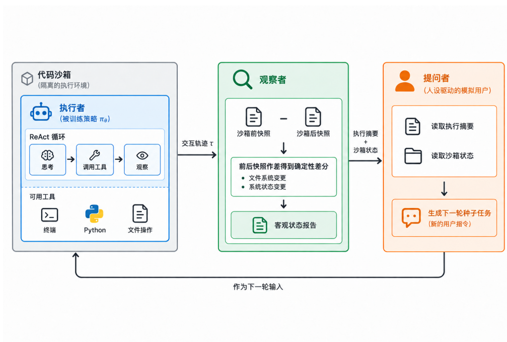
图 4.5 多智能体协作机制
