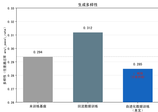
图 5.8 三个模型的生成多样性（任意通过率 any_pass_rate ）
