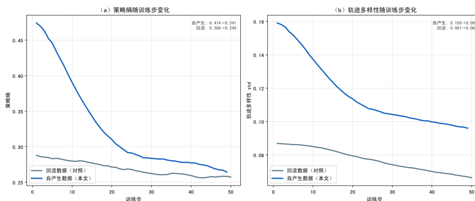
图 6.5 策略熵与轨迹多样性 std 随训练步的变化（EMA 平滑）
