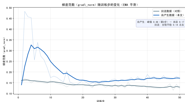
图 6.6 梯度范数 (grad_norm) 随训练步的变化
