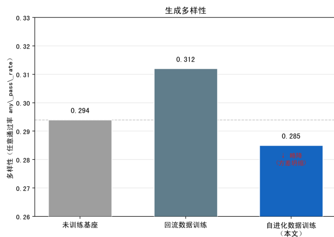
图 6.8 三个模型的生成多样性（任意通过率 any_pass_rate ）
