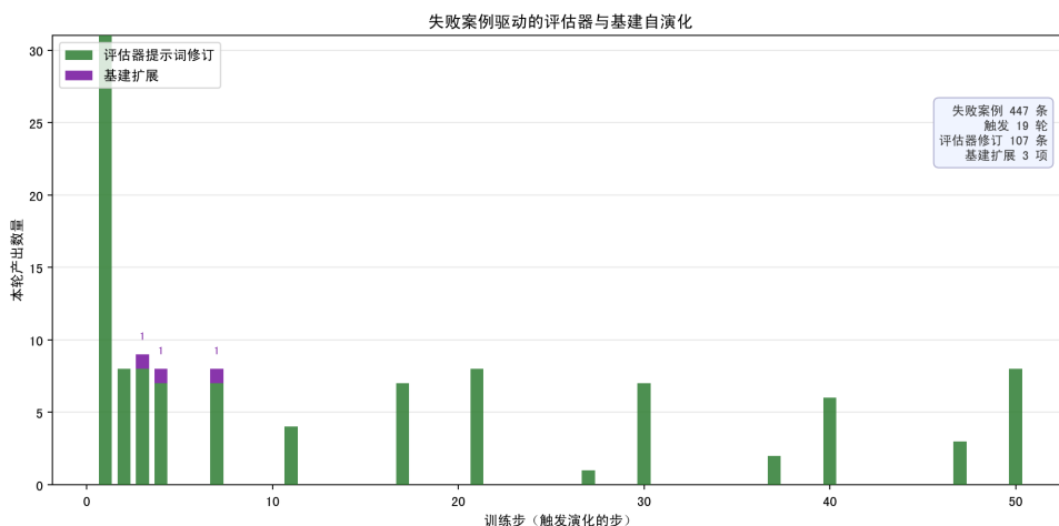
图 6.4 失败案例驱动的评价器与基建自演化时间线
