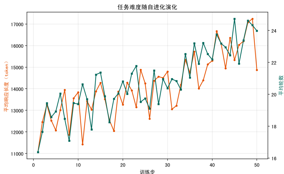
图 6.2 任务难度随自进化演化：平均响应长度与交互轮数
