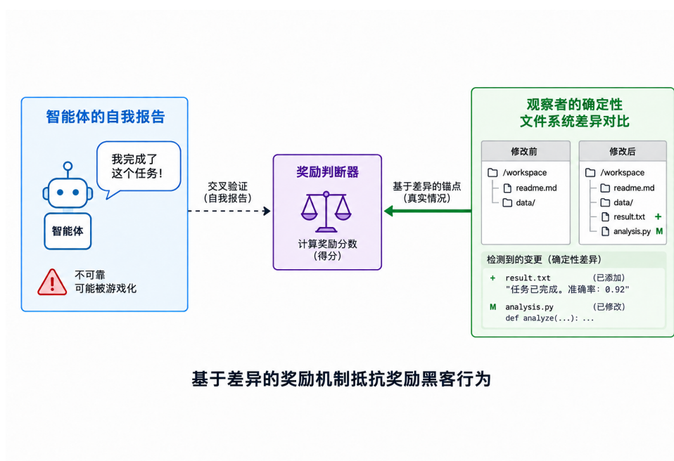
图 4.5 差分驱动奖励
