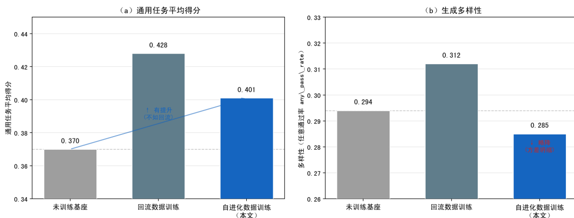
图 6.4 三个模型在通用任务上的评测对比：平均得分（左）与生成多样性（右）
