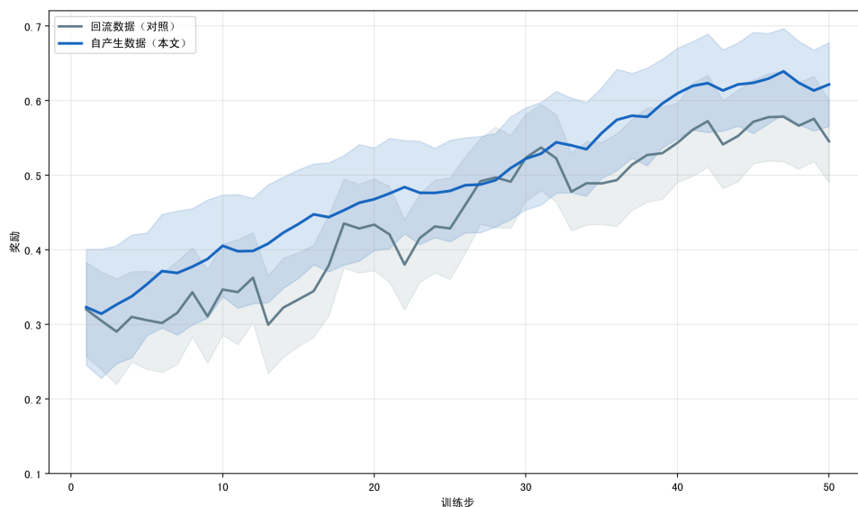
图 6.3 自产生数据（本文）与回流数据（对照）训练的奖励对比（EMA 平滑，阴影为组内奖励标准差）
