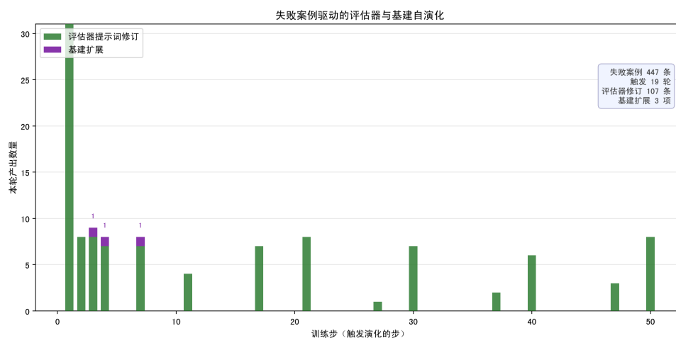
图 5.3 失败案例驱动的评估器与基建自演化时间线
