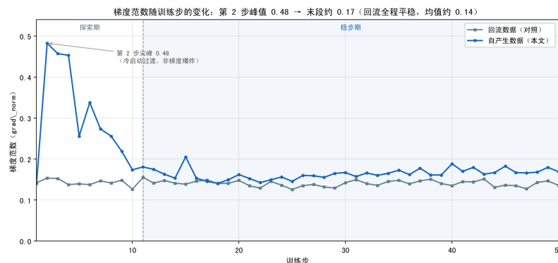
图 5.5 梯度范数 (grad_norm) 随训练步的变化 (逐步原始值)
