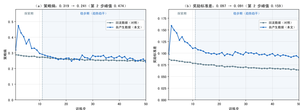
图 5.4 策略熵与奖励标准差随训练步的变化（逐步原始值）
