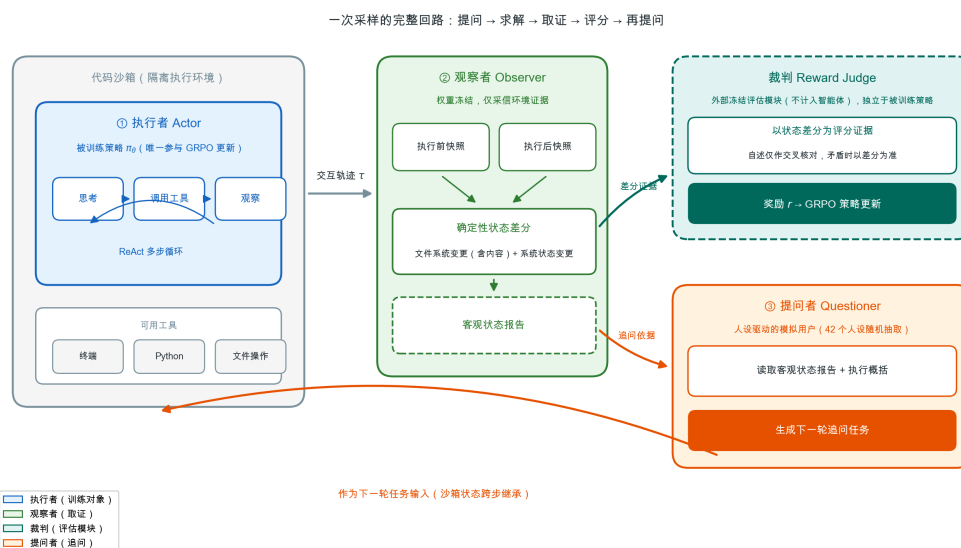
图 4.6 多智能体协作机制：三智能体与裁判的分工及一次采样的完整回路
