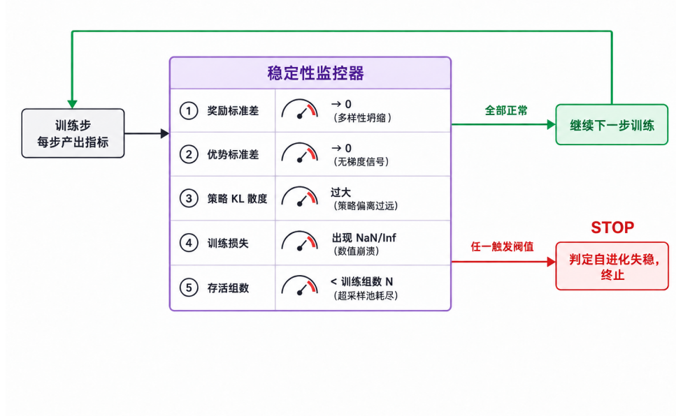
图 4.7 自进化稳定性控制：五项监控指标与自动终止判据
