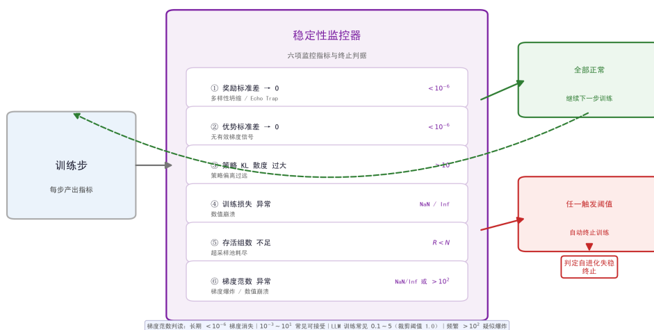
图 4.10 自进化稳定性控制：六项监控指标与自动终止判据
