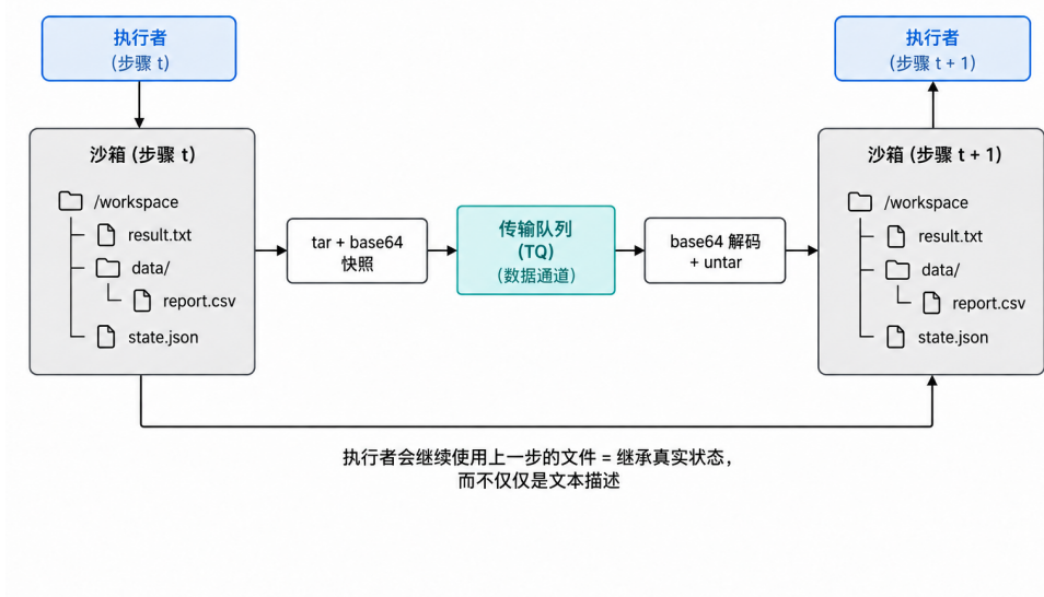
图 5.3 沙箱状态继承机制
