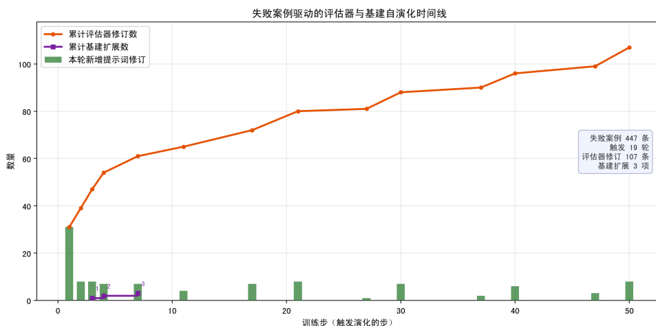
图 6.4 失败案例驱动的评估器与基建自演化时间线
