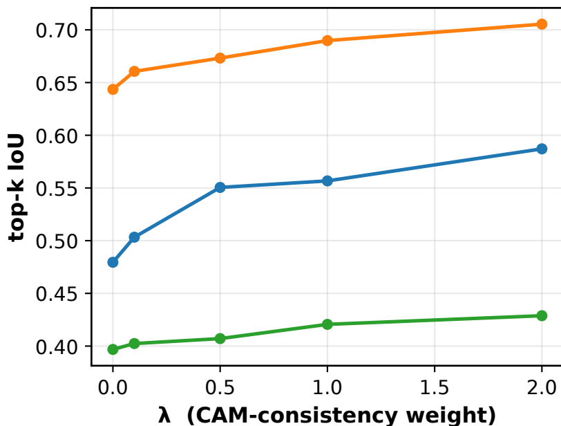
EfficientNetV2-S
