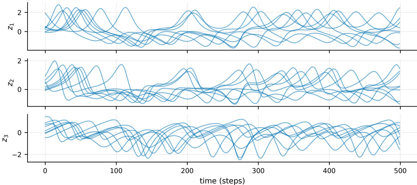
Latent trajectories — EXP-0044 (test split) (n=8 trajectories, d=3)
