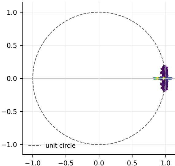
Latent Jacobian eigenvalues — EXP-0353 \max|\lambda|=1.095 ; 289/768 outside unit circle
