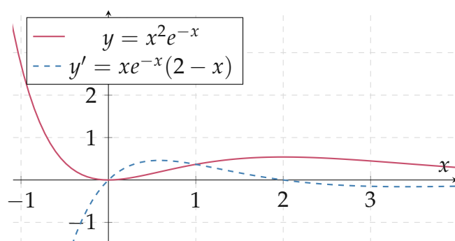
图 12.2: 函数 y = x^2 e^{-x} 及其导函数
