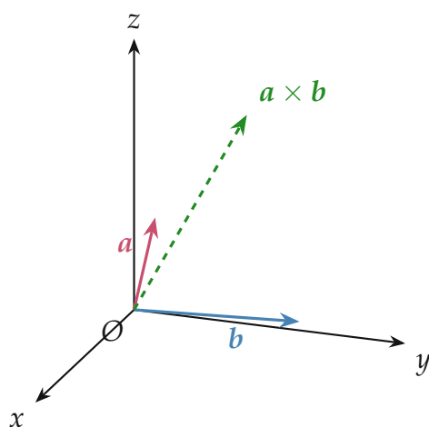
图 12.1: 向量叉积的几何意义
