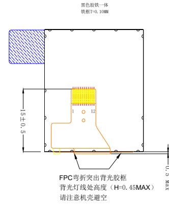
FPC弯折示意图 FPC展开出货
