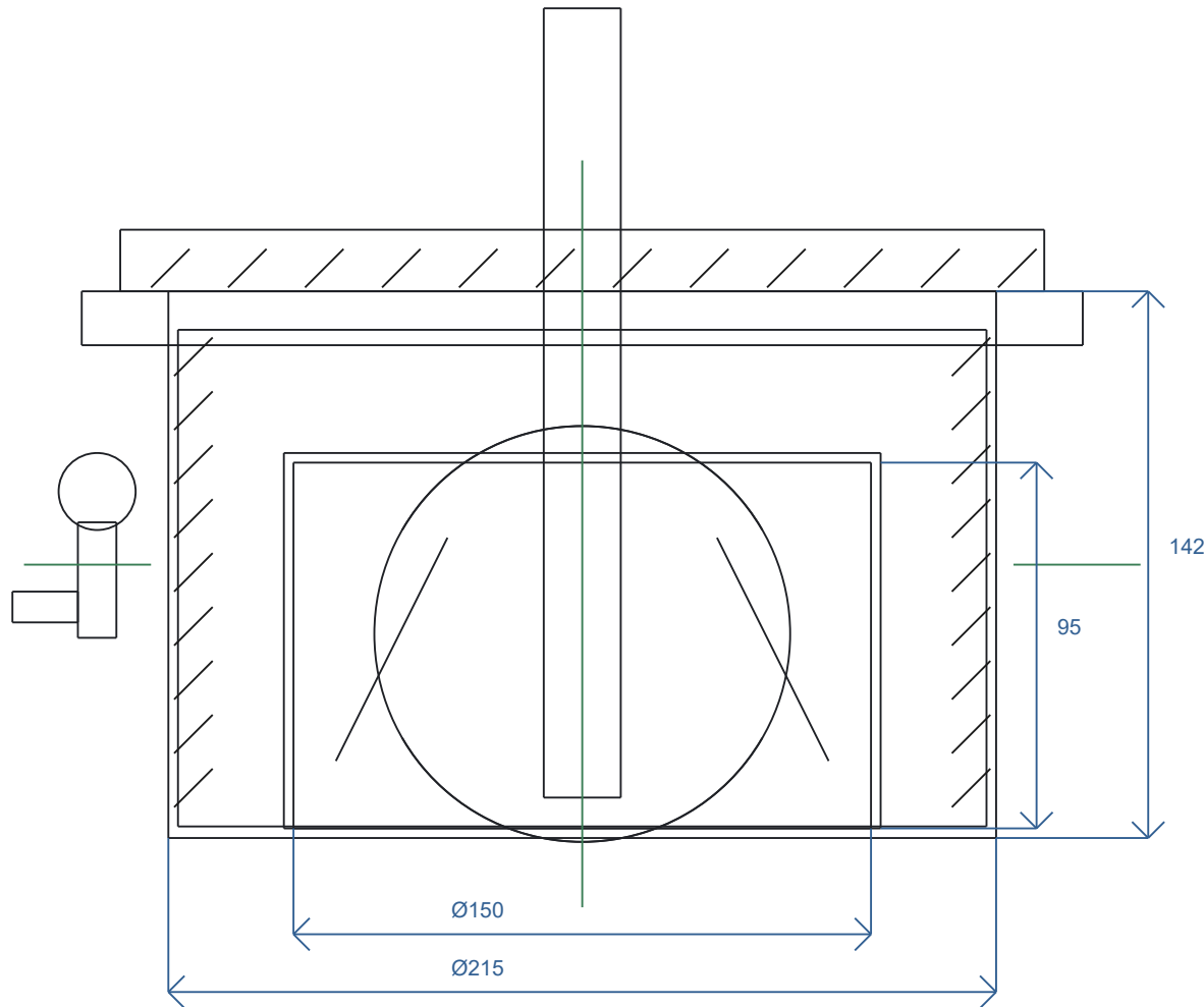
РАЗРЕЗ А-А
