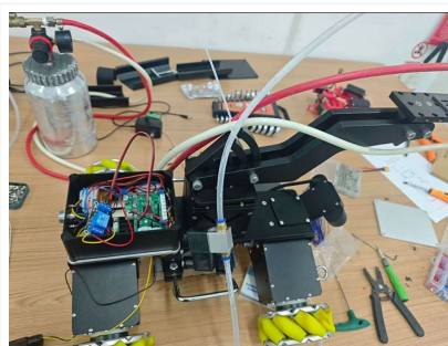
机器人本体整体组装与模块集成
