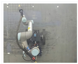
机械臂与底盘集成测试
