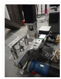
打磨执行机构调试
