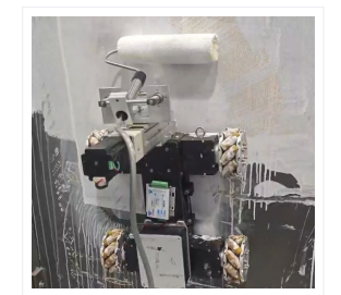
立面自动涂刷测试
