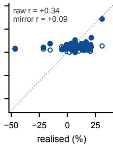
(d) Moirai-1.1
