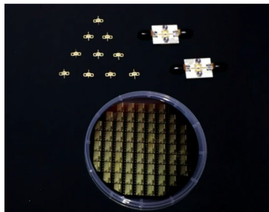
氮化镓微波二极管晶圆、器件、模块
