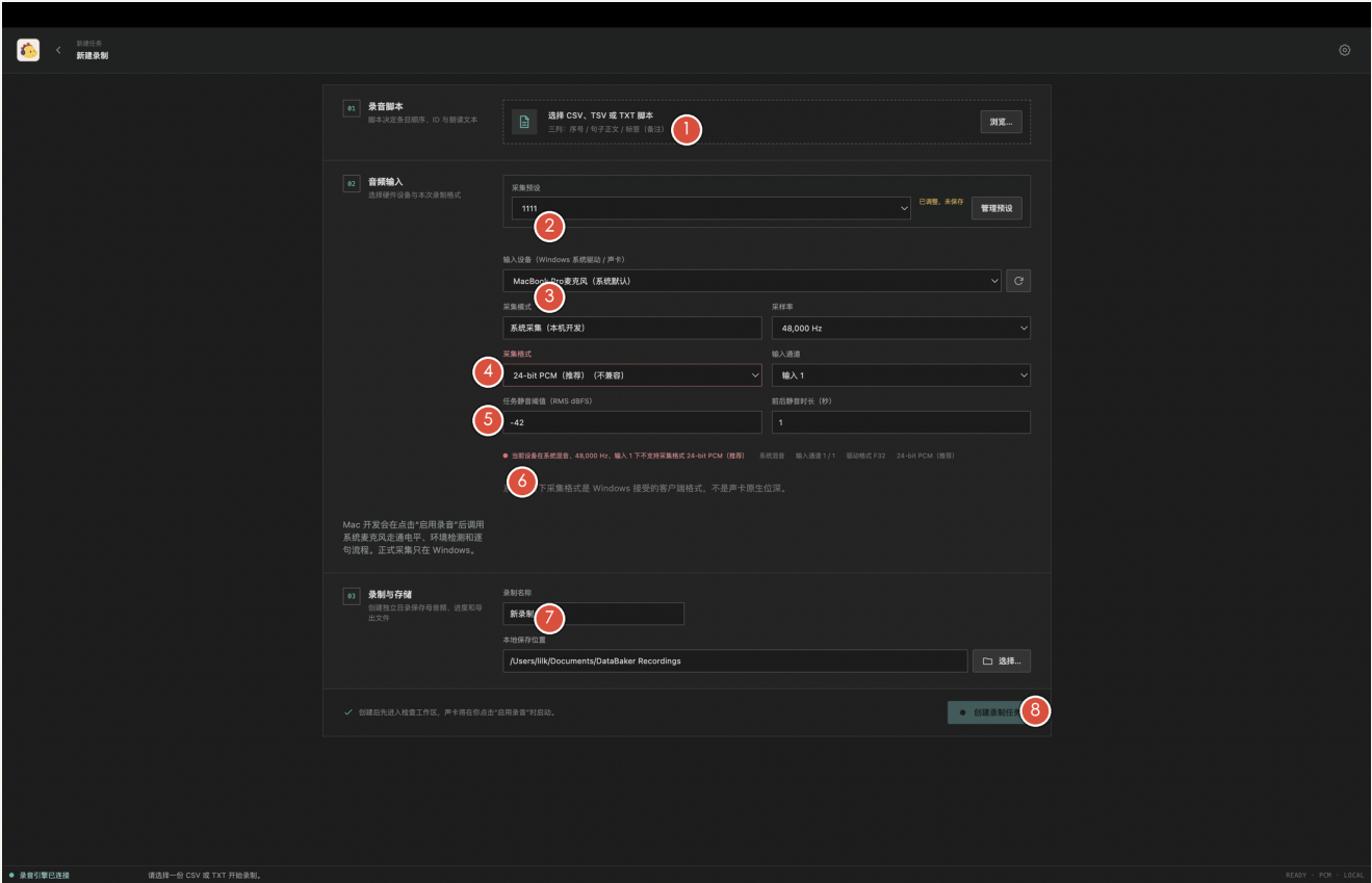
图 3 新建录制
