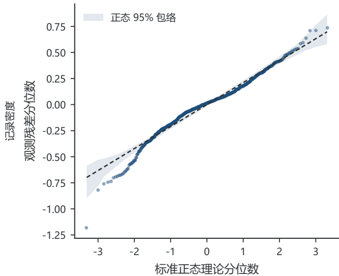
正态 Q-Q 诊断
