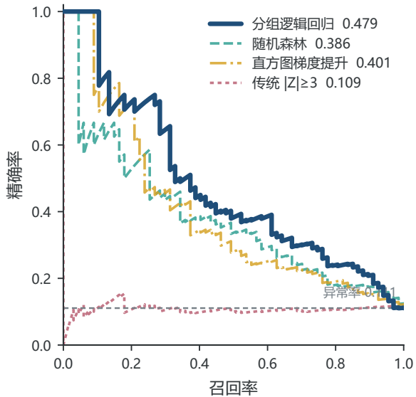
b PR 曲线 · 图例为 AP
