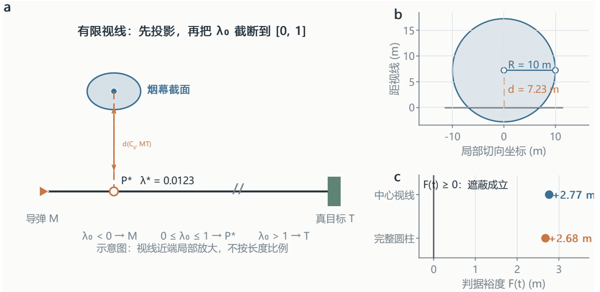
图2 有限视线判据的三层证据。A 为有限线段及最近点的非比例示意，B 为 t = 8.70 s 的真实尺度局部截面，C 为同一时刻两种遮蔽口径的裕度复算；烟幕圆未被裁切。
