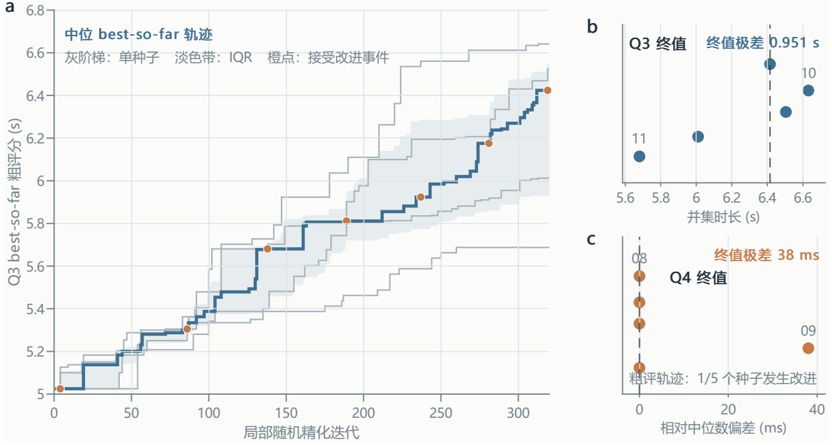
图 8 Q3、Q4 五个独立种子的事件阶梯与连续终值脊线。左侧按 best-so-far 事件前向保持，不用直线插值虚构改进；右侧只标端点极差和极端种子。
