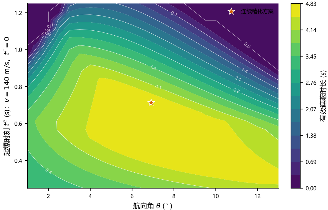
问题 2：主口径目标函数的二维剖面
