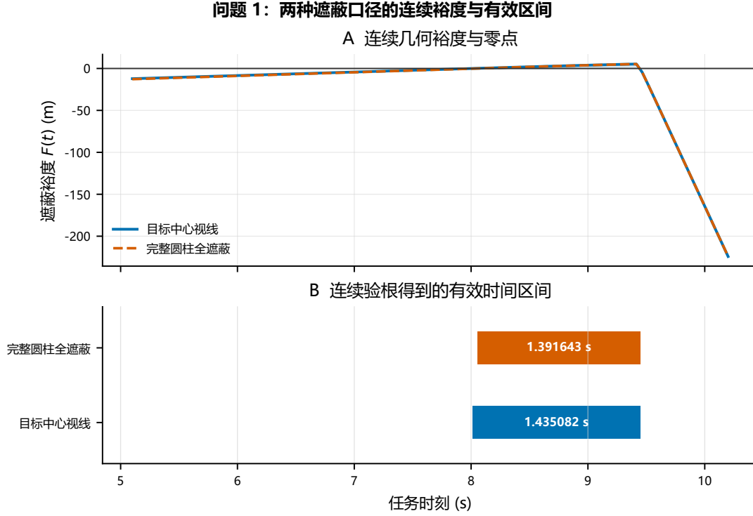
图 3 Q1 两种遮蔽口径的连续裕度与有效区间。零水平线给出连续进入和退出边界；圆柱口径的进入时刻较晚。
