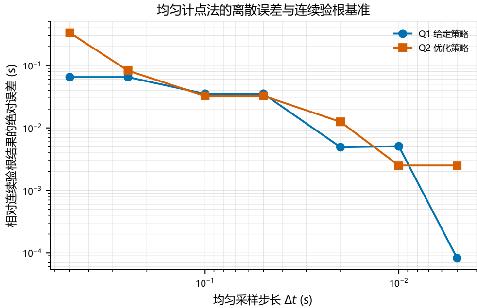
图 13 Q1、Q2 均匀计点法相对连续验根的绝对误差。横轴为扫描步长，纵轴为时长误差；连续值作为比较基准。
