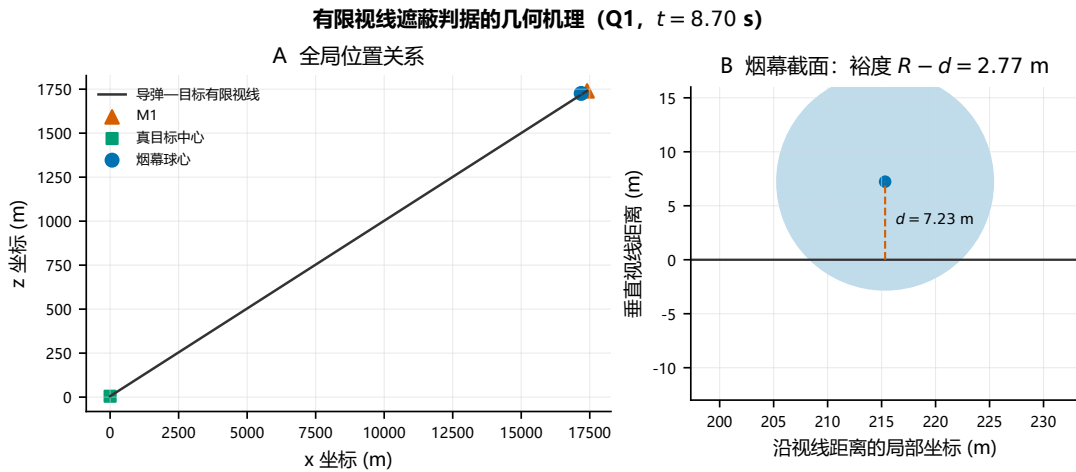
图2 有限视线几何与烟幕截面的尺度关系。烟幕是否有效由球心到导弹-目标有限线段的距离决定。
