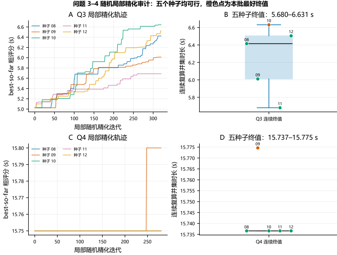
图 8 Q3、Q4 五个独立种子的随机局部精化轨迹与连续复算终值分布。Q3 离散明显，Q4 多数种子停在同一平台；所有运行的最大约束违反量均为 0。
