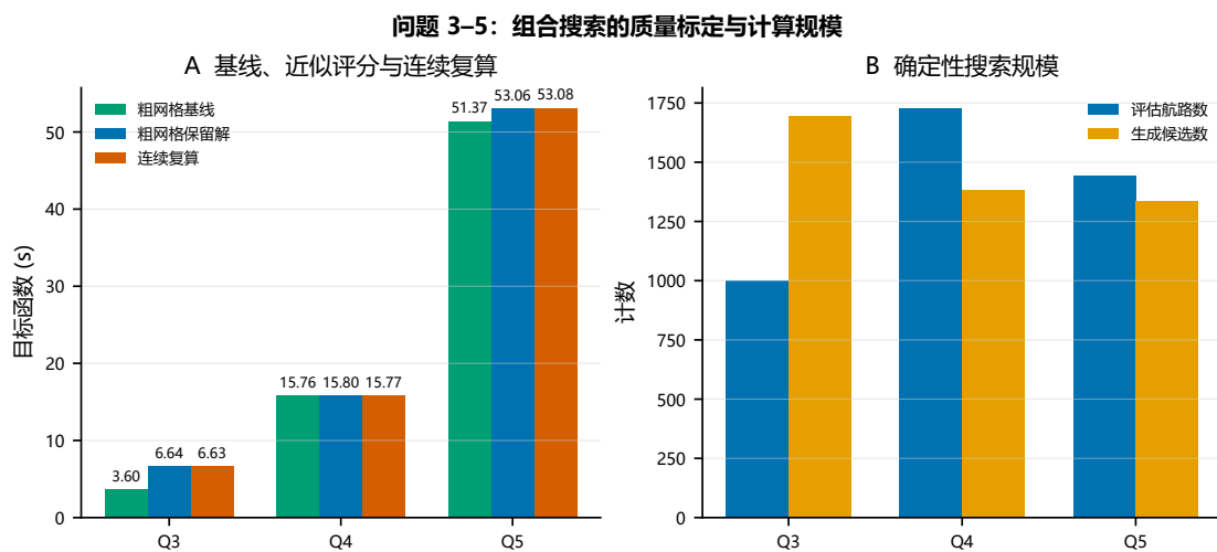
图 9 Q3–Q5 的快速基线、候选粗评分、连续复算和搜索规模。不同评分层只用于展示数值迁移；连续复算值才是终稿值。
