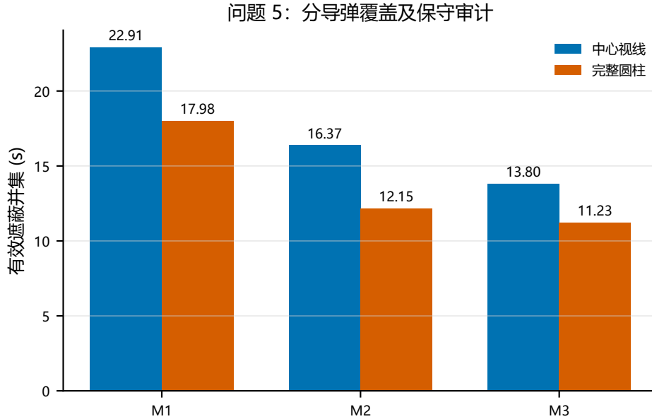
图 12 Q5 同一策略在目标中心视线与完整圆柱口径下的分导弹配对审计。柱上数值来自同一次策略复算。
