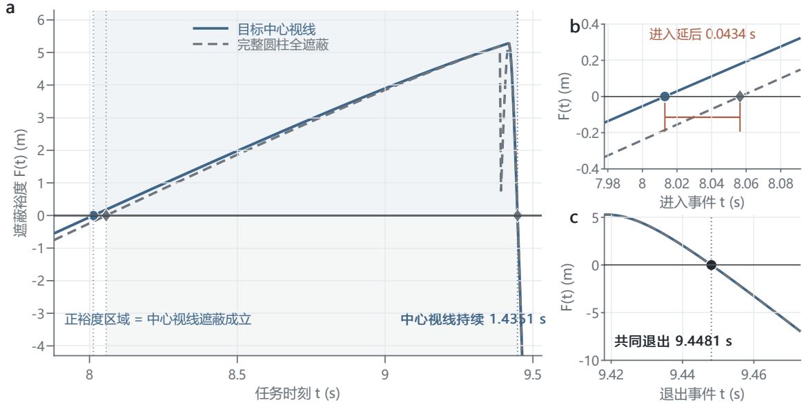
图3 问题一零点邻域的遮蔽裕度与连续边界检验。A 给出两种判据的裕度曲线及进入、退出边界，B 表示圆柱整体遮蔽判据相对中心视线判据的进入延迟 0.0434 s，C 放大两种判据的共同退出边界。
