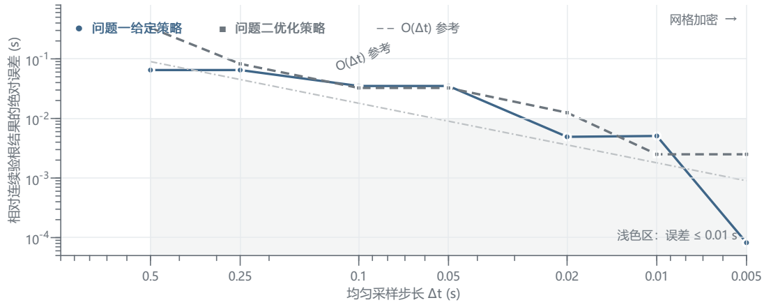
图 9 均匀时间网格相对连续求根结果的绝对误差。横轴由左至右表示时间步长减小，虚线为 O(\Delta t) 参考线，浅色区域表示误差不超过 0.01 s。
