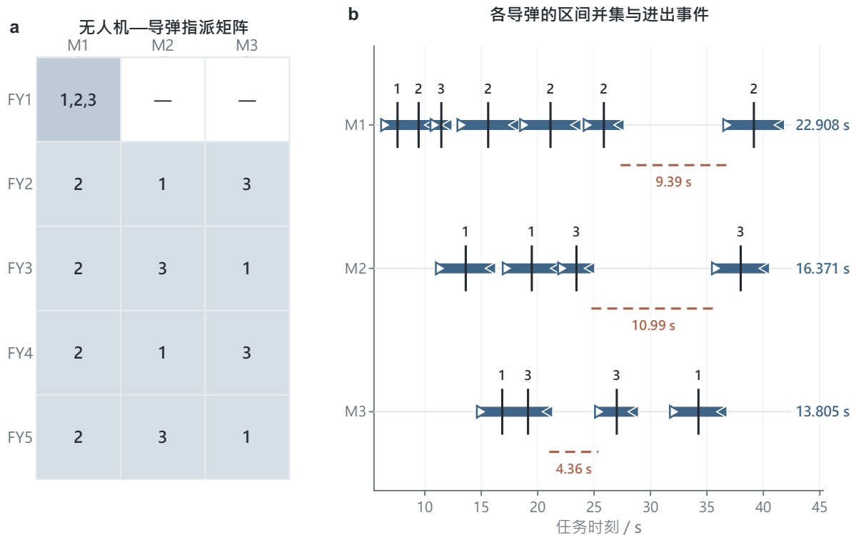
图 8 问题五的无人机—导弹指派与区间并集。左图格内数字为各无人机指派给 M1–M3 的烟幕弹序号；右图以进入、退出事件给出三枚导弹的精确区间并集，暖色虚线标出最大内部空窗。
