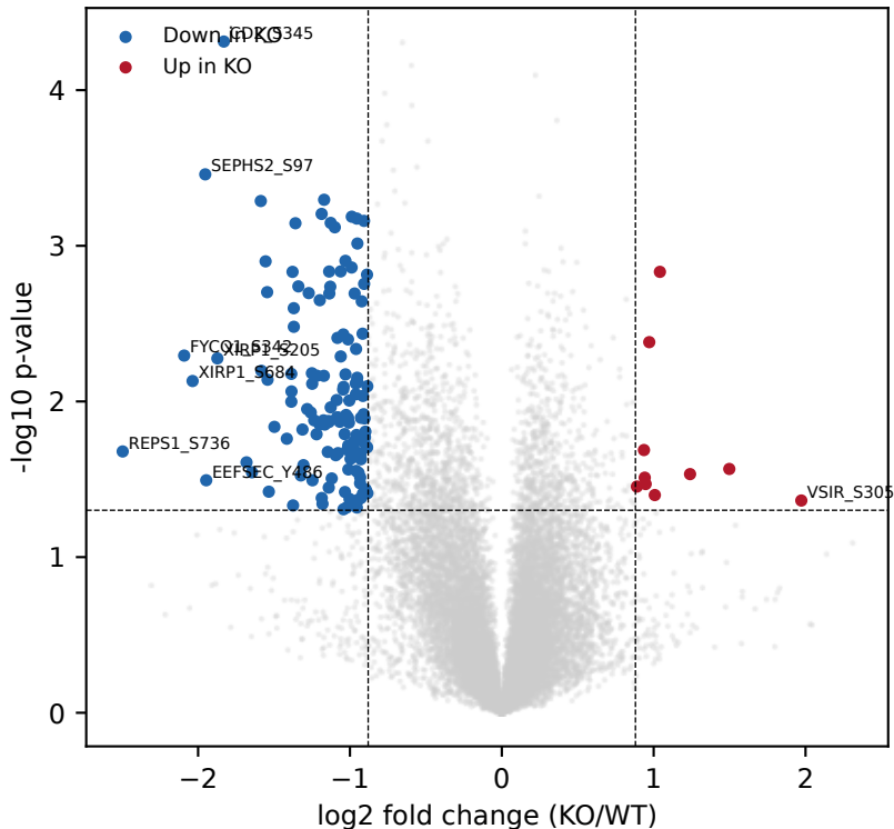
CD2-KO vs WT, 30min (n=16608)
