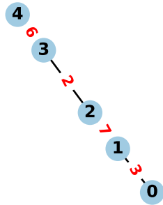
Path P_5 ( N=5 , E=4 )
