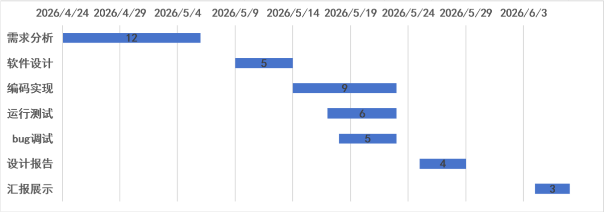
图 1: 项目甘特图
