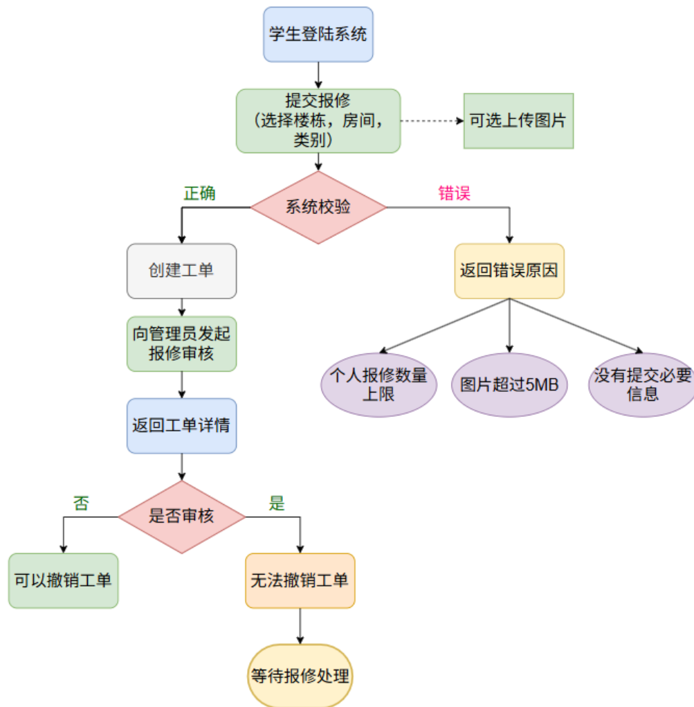
图 6: 学生报修业务流程图
