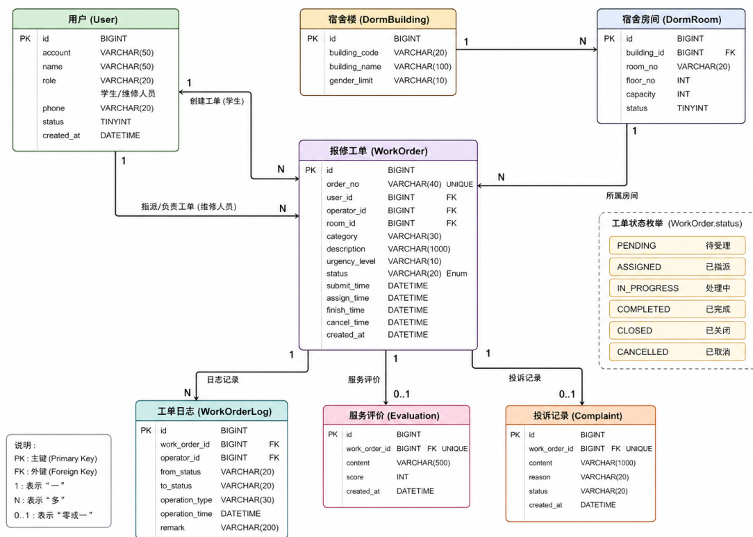
图 15: 系统实体联系图 (E-R 图)
