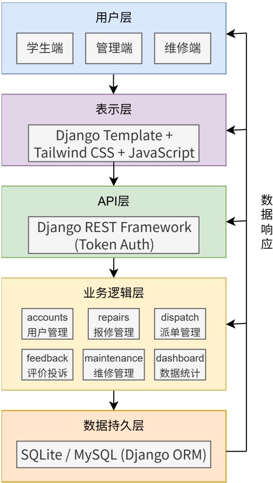
图 2: 系统总体逻辑架构图
