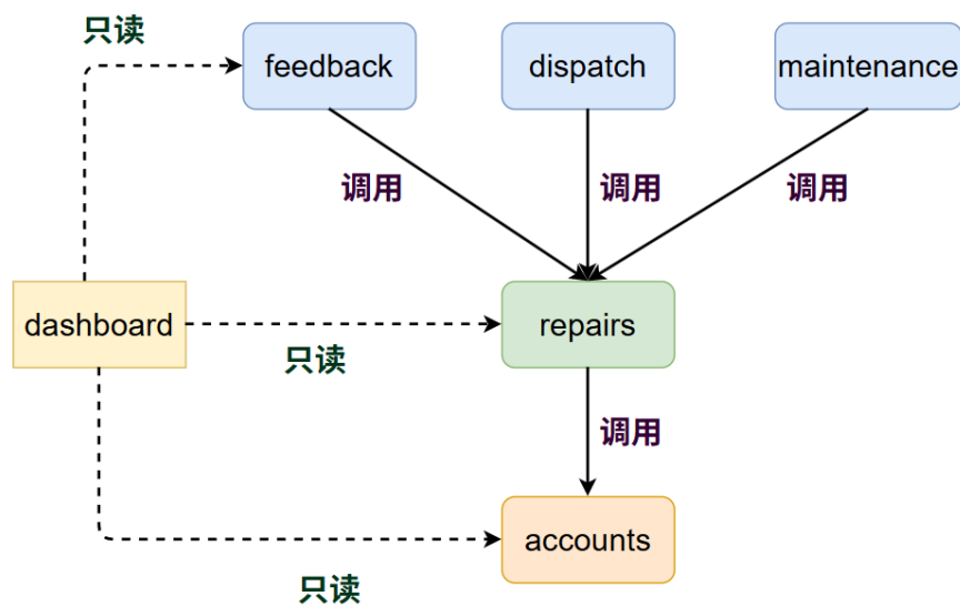
图 5: 系统模块调用关系图
