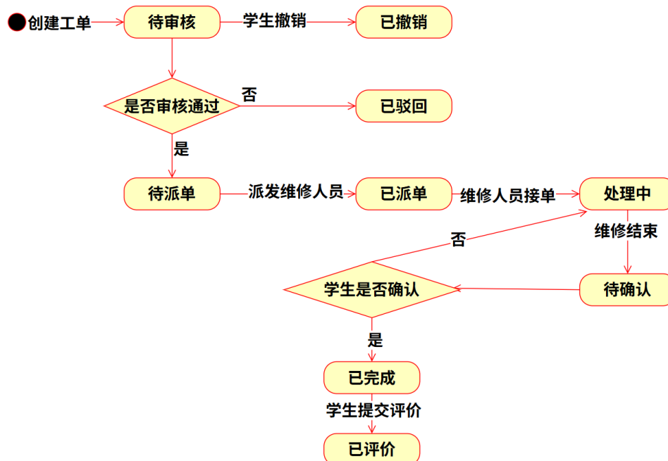
图 13: 报修工单状态图
