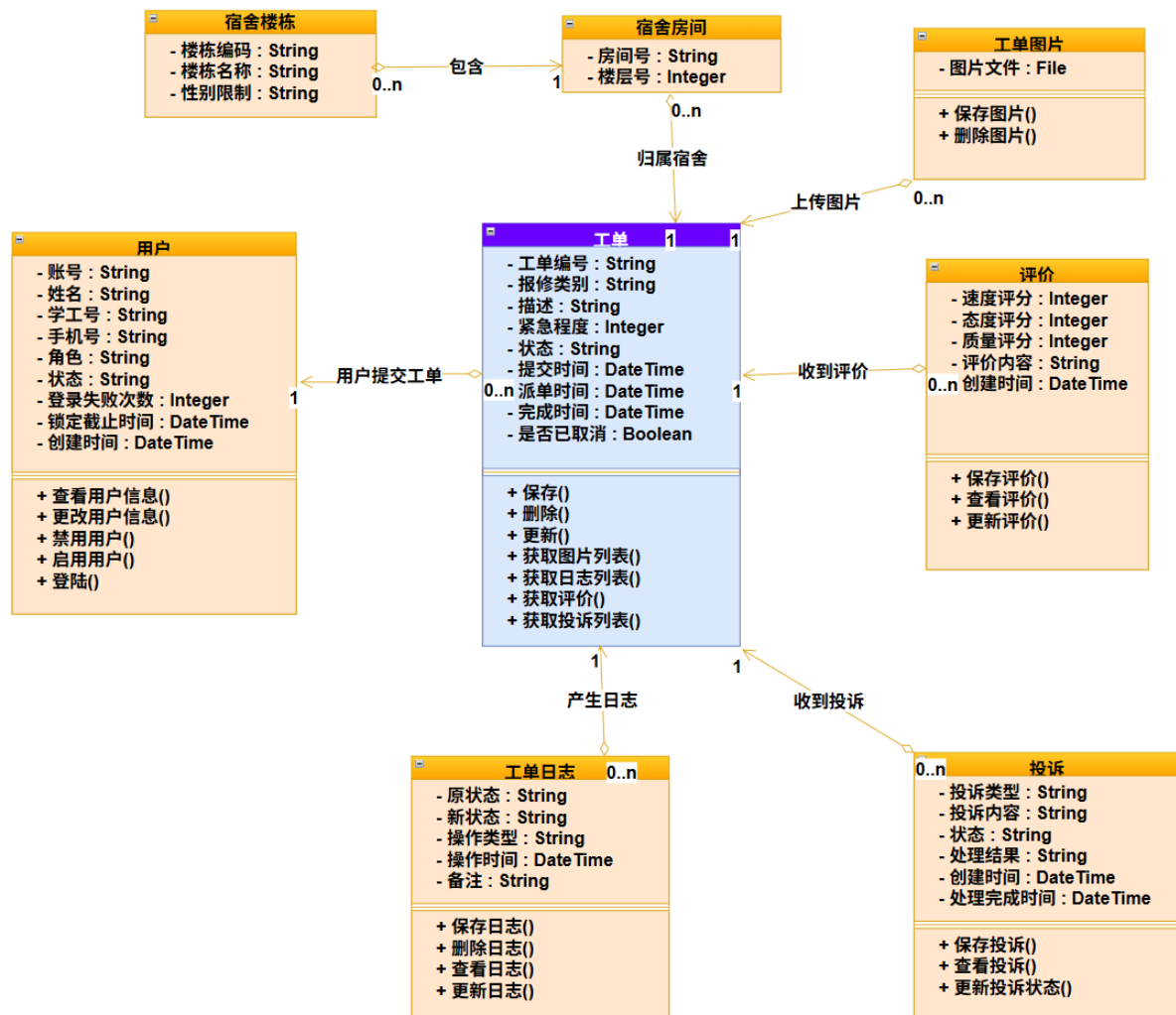
图 10: 系统核心业务类图
