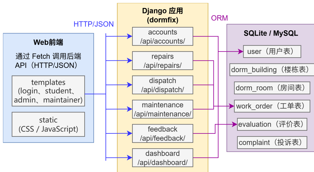
图 3: 系统整体结构图（前端、后端应用与数据库）
