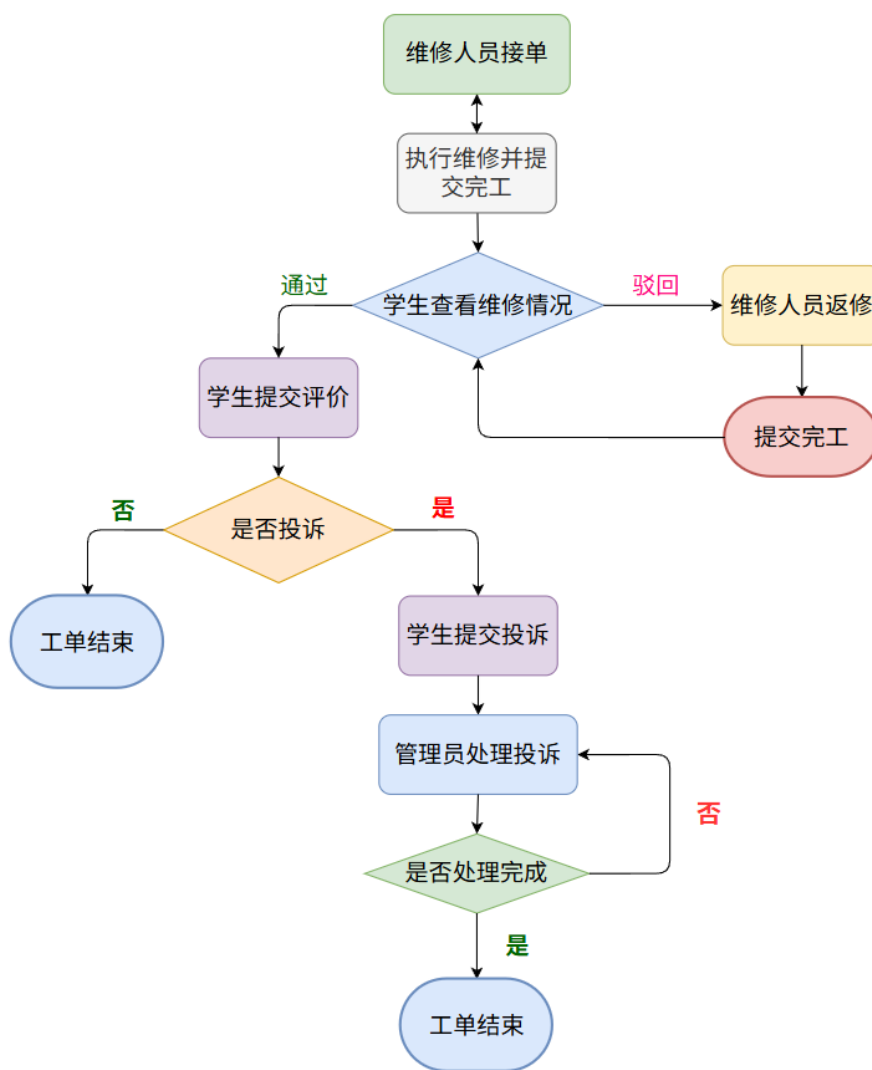
图 8: 维修处理与学生确认业务流程图
