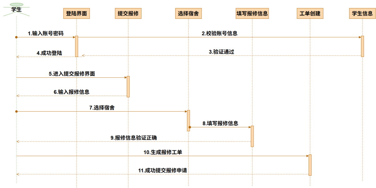
图 11: 提交报修申请顺序图 (UC002)
