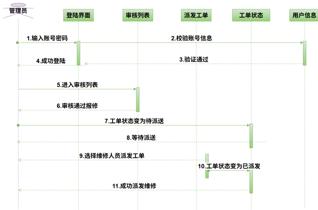
图 12: 派发维修任务顺序图 (UC006)
