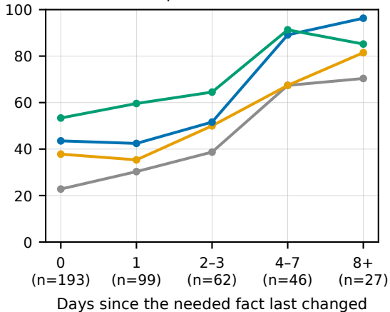
DeepSeek-V4-Flash
