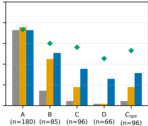
DeepSeek-V4-Flash
