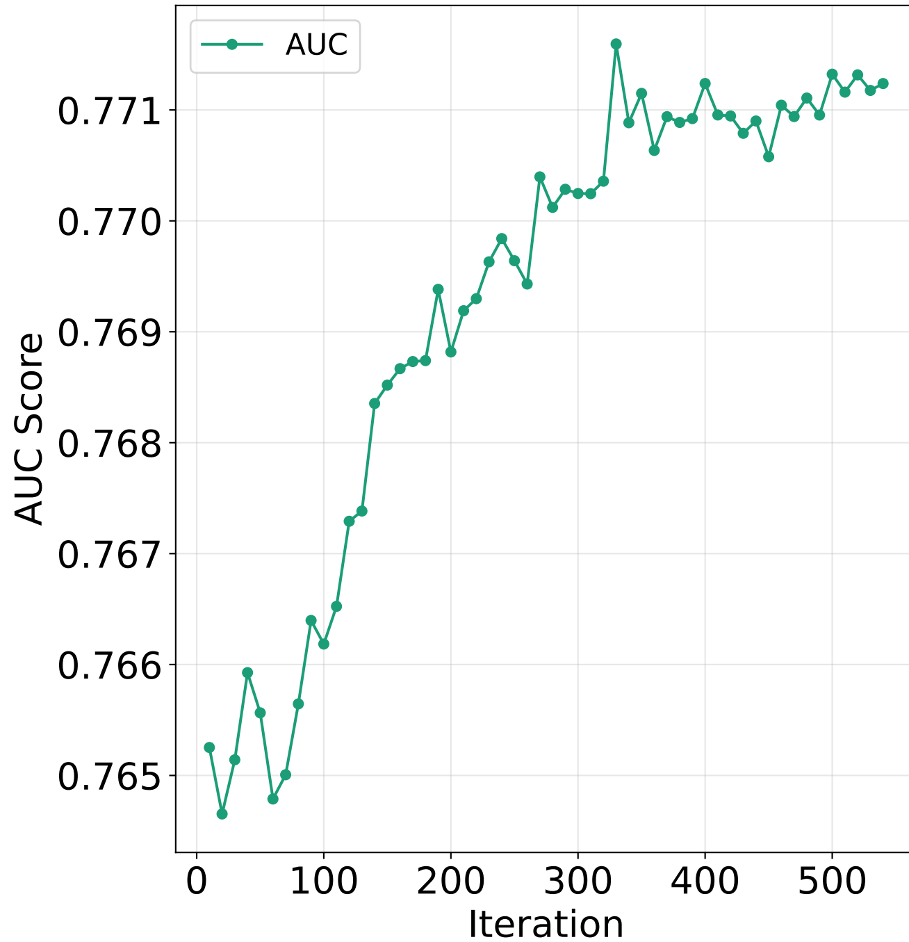
AUC Metrics
