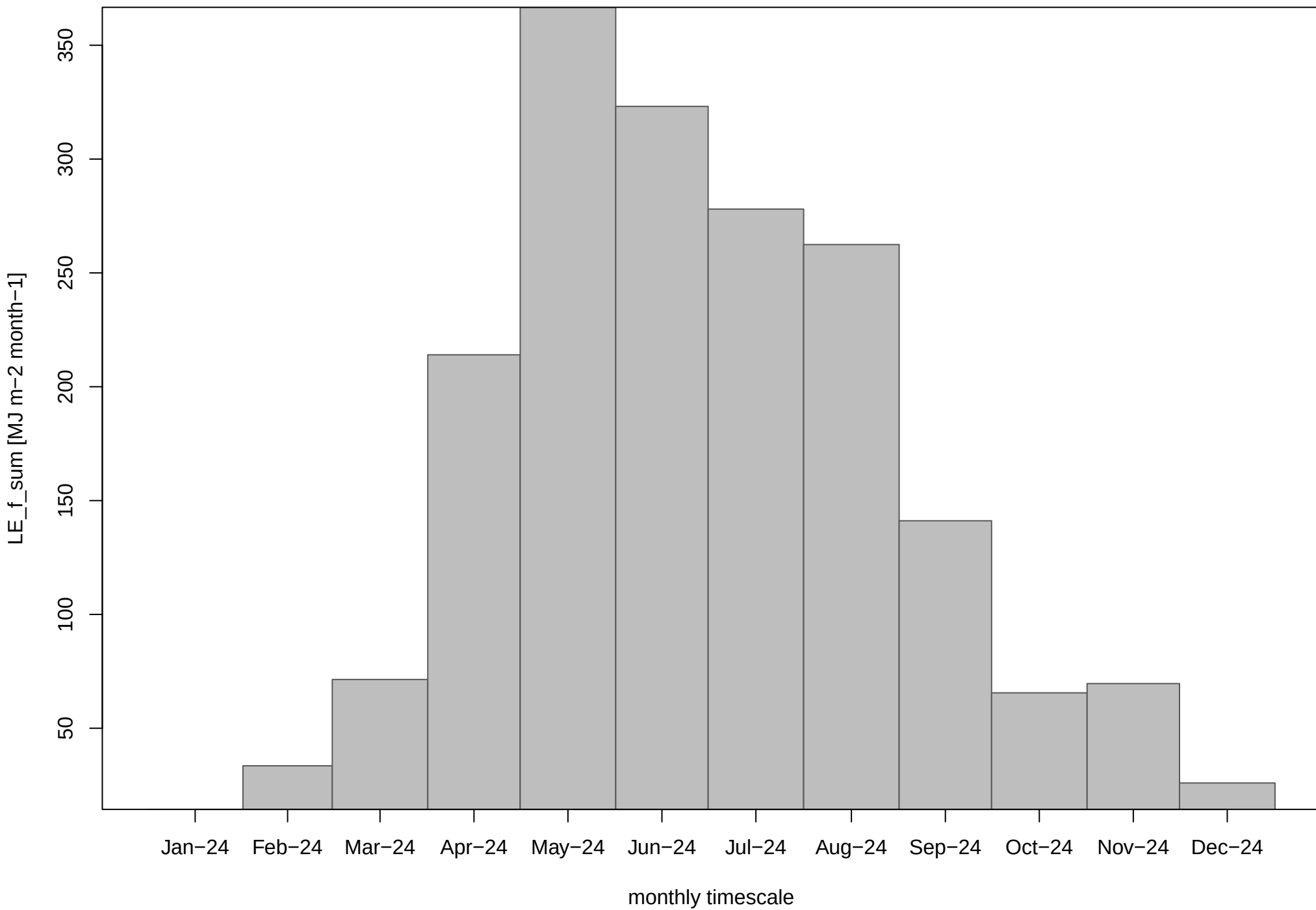
LE_f_sum
