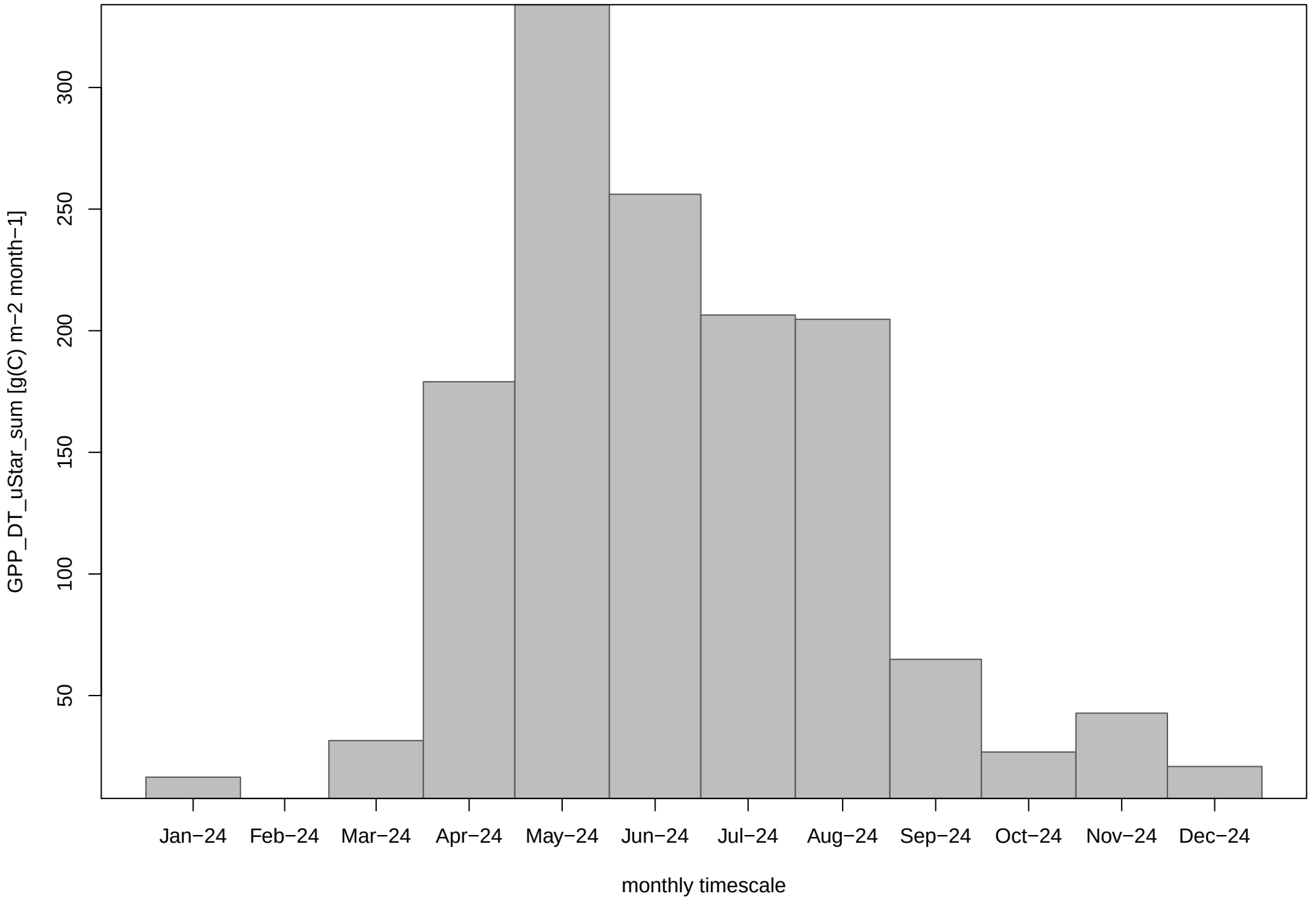
GPP_DT_uStar_sum
