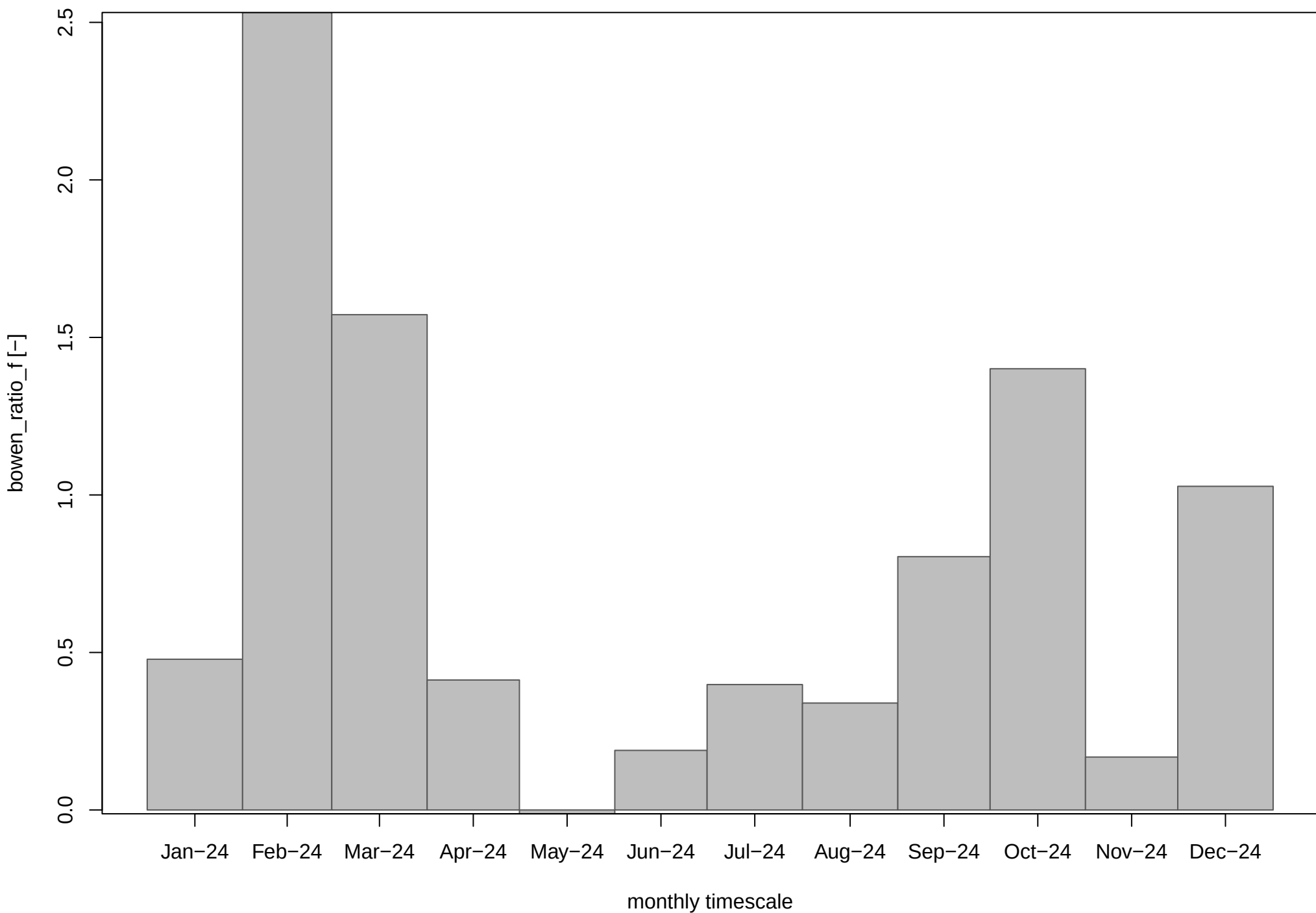
bowen_ratio_f
