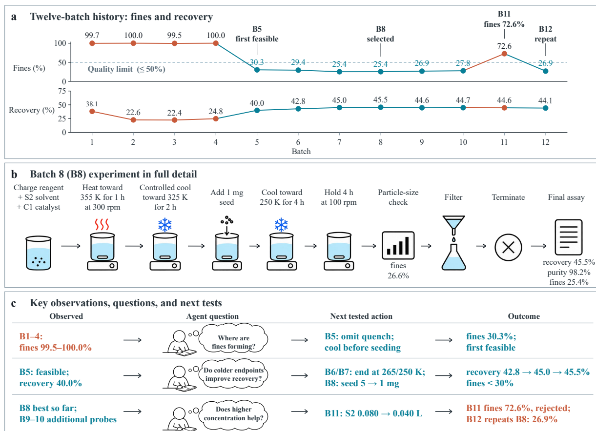
图 2 一场完整的自主结晶研究。a，事后选取的 W04/MisIndexed 会话中全部 12 批来源实验。数值为记录的最终检测结果；青色表示满足质量约束，赭色表示失败。虚线表示 50% 的细晶比例上限。第 5 批首次可行，第 8 批最终被封存为推荐方案，第 11 批违反细晶约束，第 12 批重复所选配方。b，来源第 8 批的全部 12 次操作调用，归为 10 个可见阶段。中间粒径检查读数为 26.6% 细晶，最终检测为 25.4%。温度表示请求的目标值，而非实测温度轨迹。独立复测使用封存的第 8 批配方和不同的观测随机种子。c，三组“观测、后续行动、结果”序列。问题由作者根据操作记录重建，并非模型当时的原话；K1 在实验序列结束后撰写。第 5 批同时改变多个工艺条件，因此无法单独识别省略终止反应操作（quench）的作用。回收率不计入晶种质量。可行性要求纯度至少 80%、细晶比例至多 50%，且存在颗粒；细晶指小于 20 微米的颗粒。本例用于展示研究过程，不用于估计总体发生频率。
