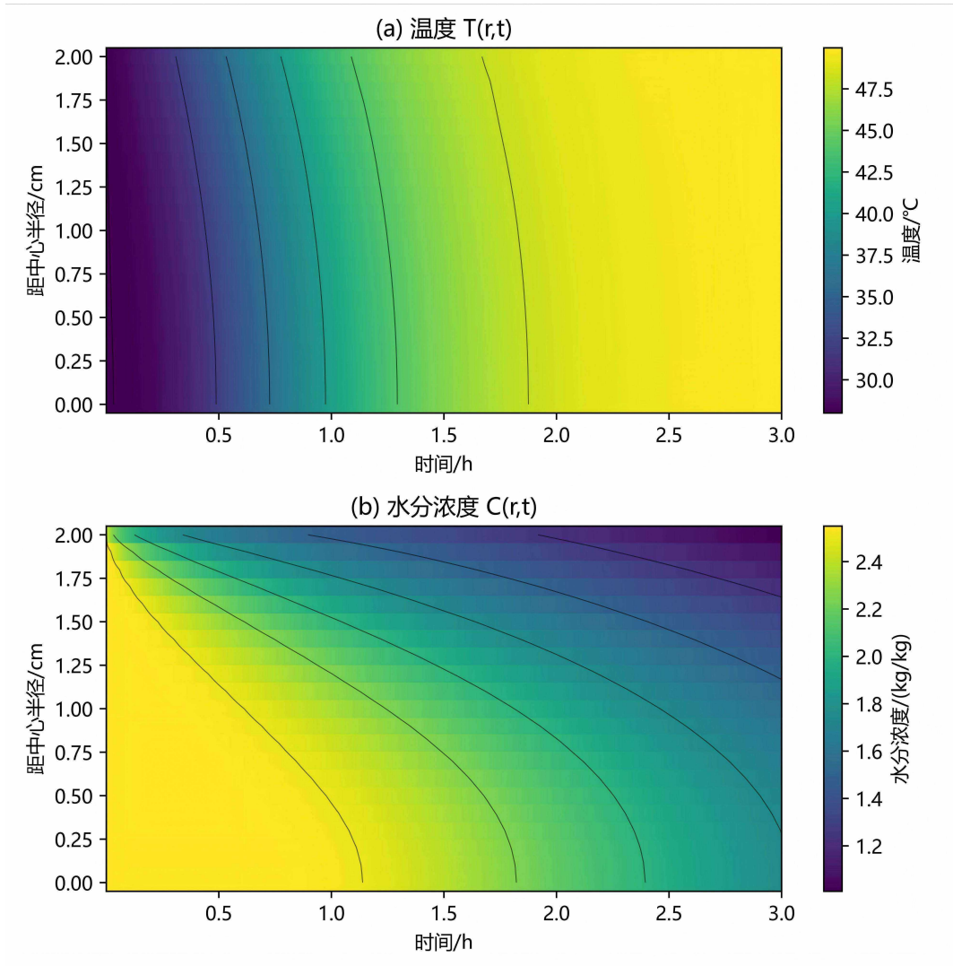
图 5 变物性热湿耦合条件下温度与水分浓度的时空演化。(a) 温度 T(r,t) ; (b) 水分浓度 C(r,t) ; 黑色细线为等值线。温度场约 2h 内接近烘房温度、径向梯度消失; 水分场在整个 3h 内保持明显径向梯度, 说明恒温干燥阶段受内部水分扩散控制。
