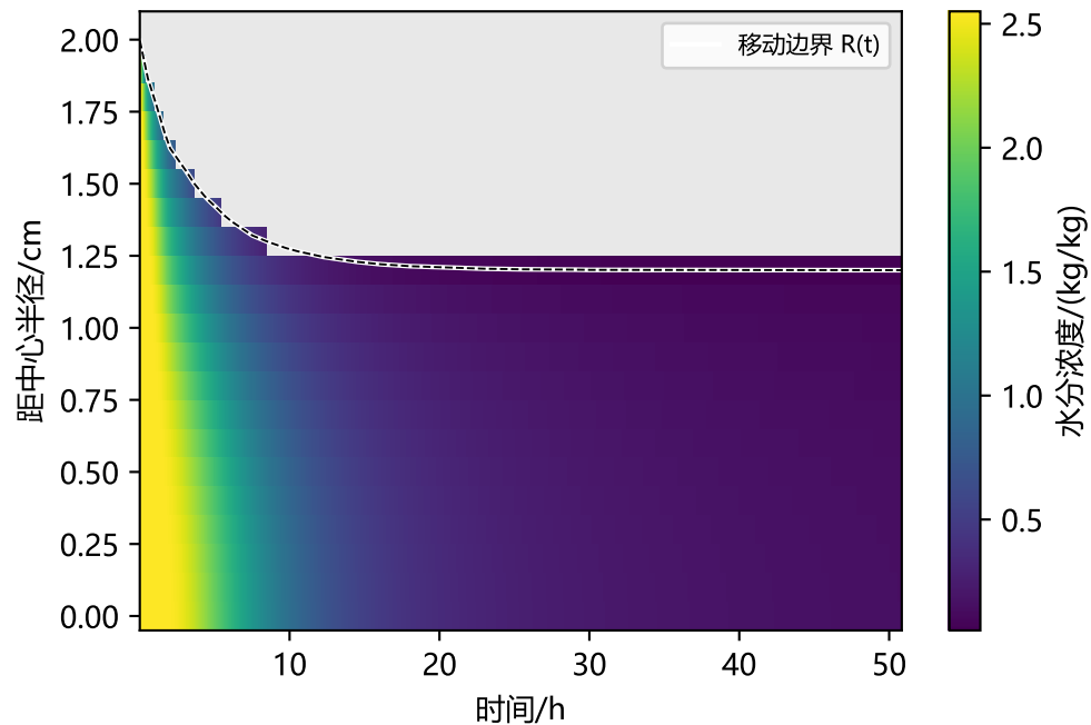
(a) 物理坐标水分演化与移动边界 (灰色=已收缩区域)
