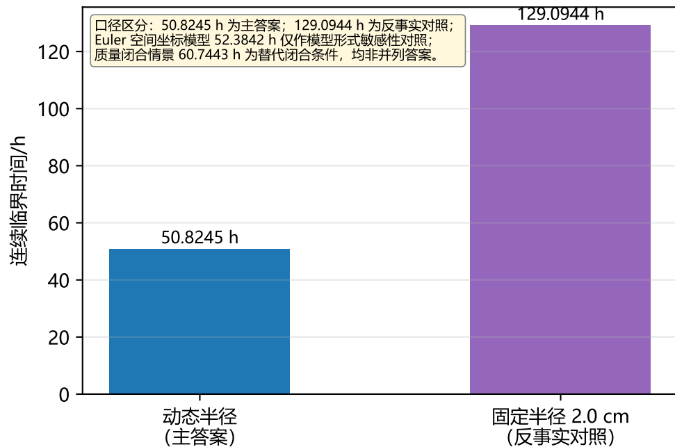
(b) 收缩作用消融对照 (缩短 78.2699 h)
