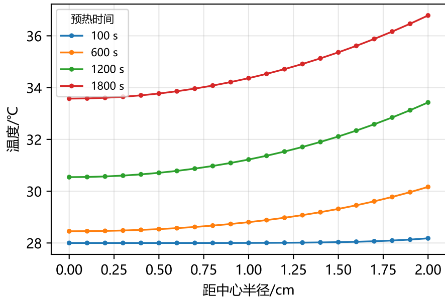
(a) 温度径向分布
