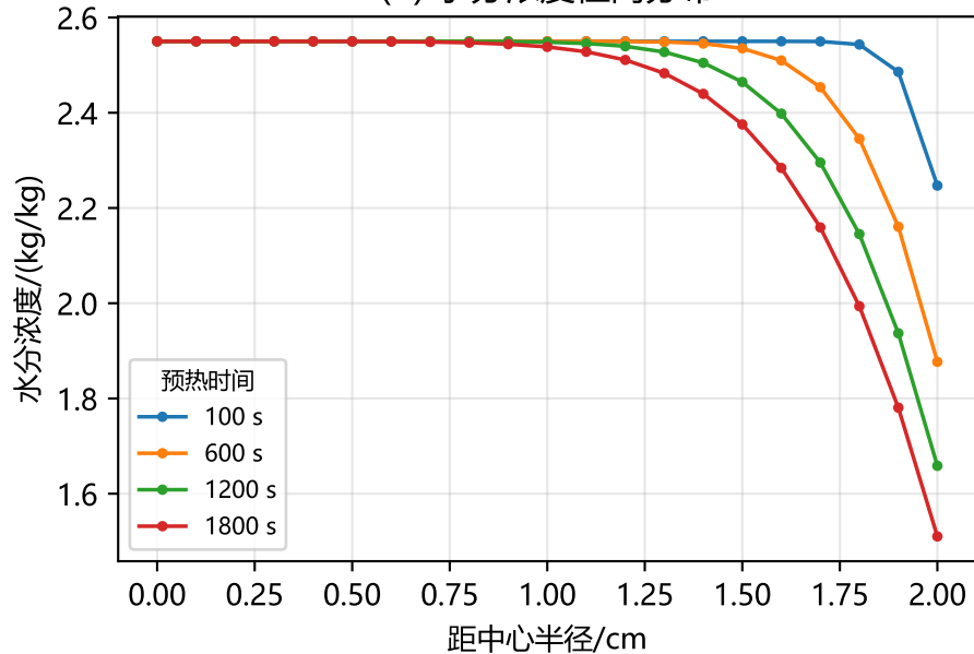
(b) 水分浓度径向分布
