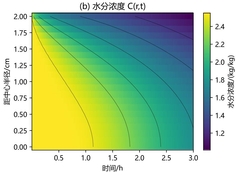
图2 变物性热湿耦合条件下温度与水分浓度的时空演化
