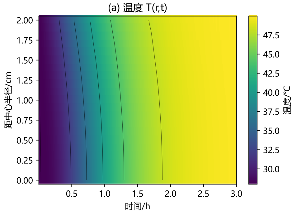
图2 变物性热湿耦合条件下温度与水分浓度的时空演化
