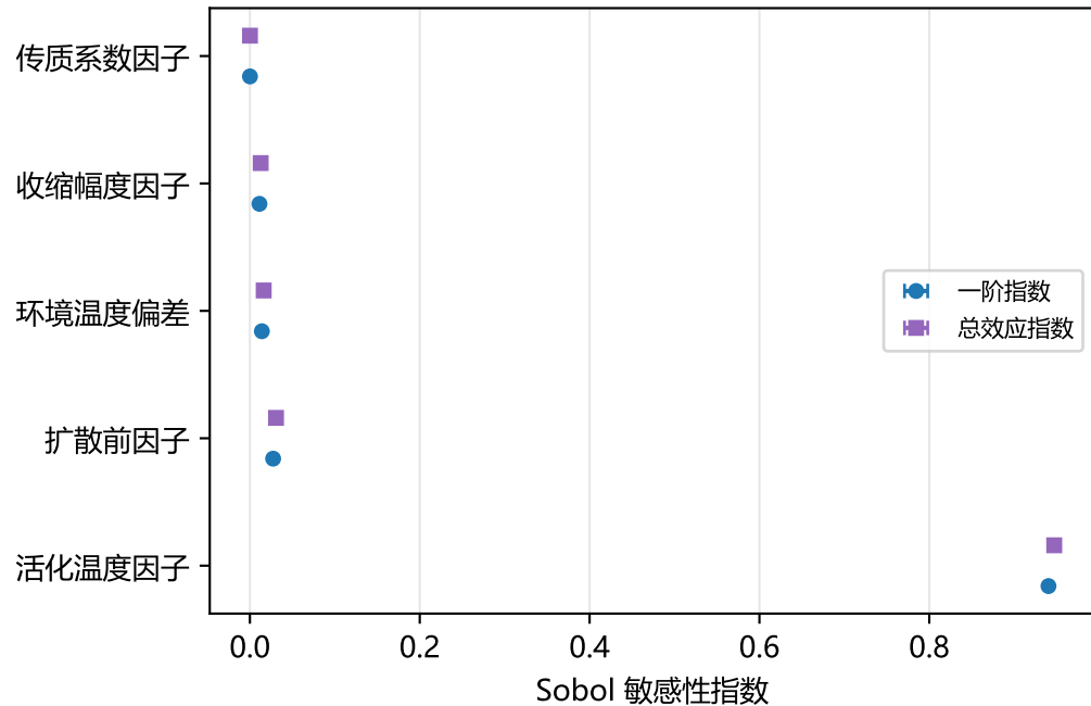
(b) 干燥时间的 Sobol 全局敏感性
